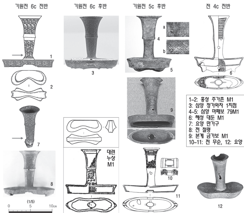
그림 4 요동(요중)지역 청동검병의 계보와 변천
