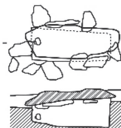
개석 II a식 (봉성 동산2호)
