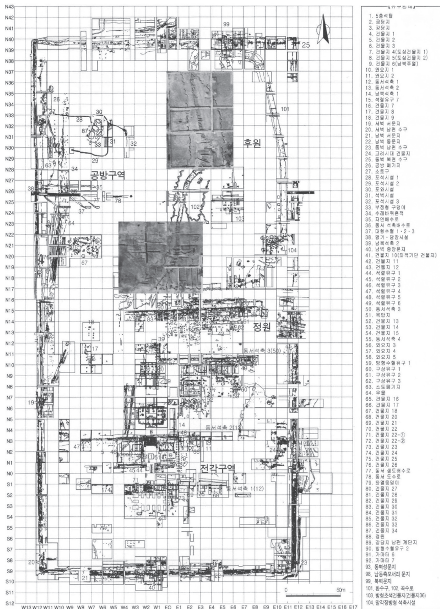
그림 13 익산 왕궁리 유적의 유구 배치도(김낙중, 2011)
