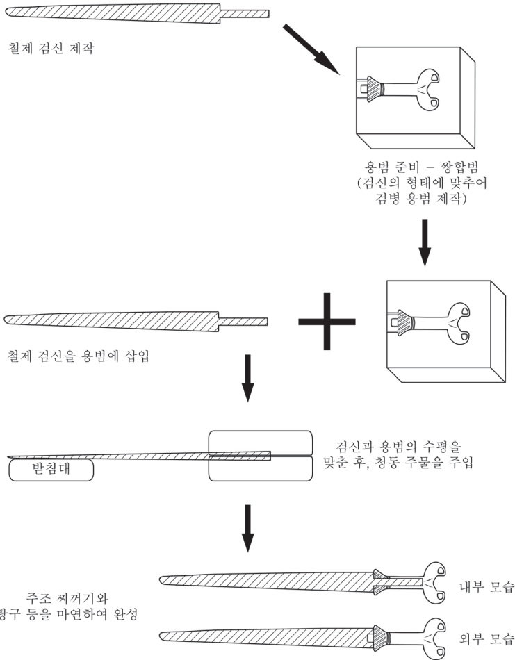
그림 6 동병철검 제작 모식도(이청규·김동일, 2013 수정 후 전제)
