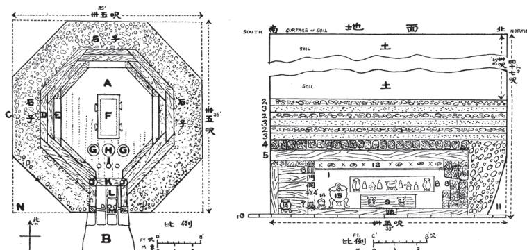
그림 6 V호묘 평·단면도(White, 1934)
