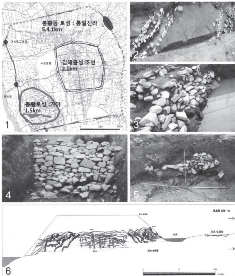
그림 2 1. 봉황토성 위치도, 2~3. 석축보강유구, 4~5. 보강 석축, 6. 모식도(심광주, 2023)
