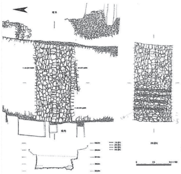
금산 백령산성 남문지(백제)
