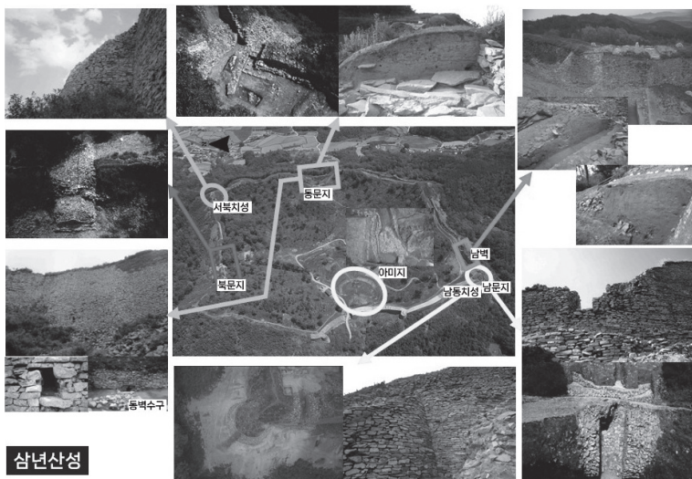
그림 7 보은 삼년산성 현황(오른쪽 위는 5세기 후반 신라 토축성벽, 이 외는 통일신라시대 이후 석축성벽)(중원문화재연구원, 2008·2009 전채 및 재편집)
