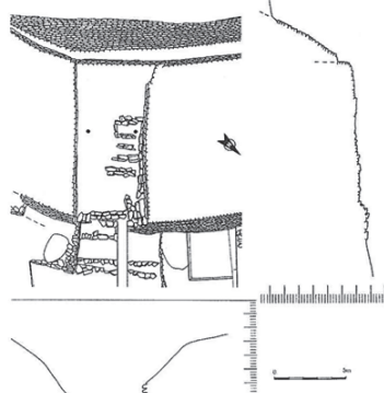
금산 백령산성 남문지(백제)
